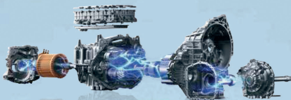
Transmisión longitudinal 2DHT
