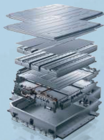
Batería Off-road CATL
